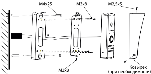
Монтаж с угловым кронштейном
