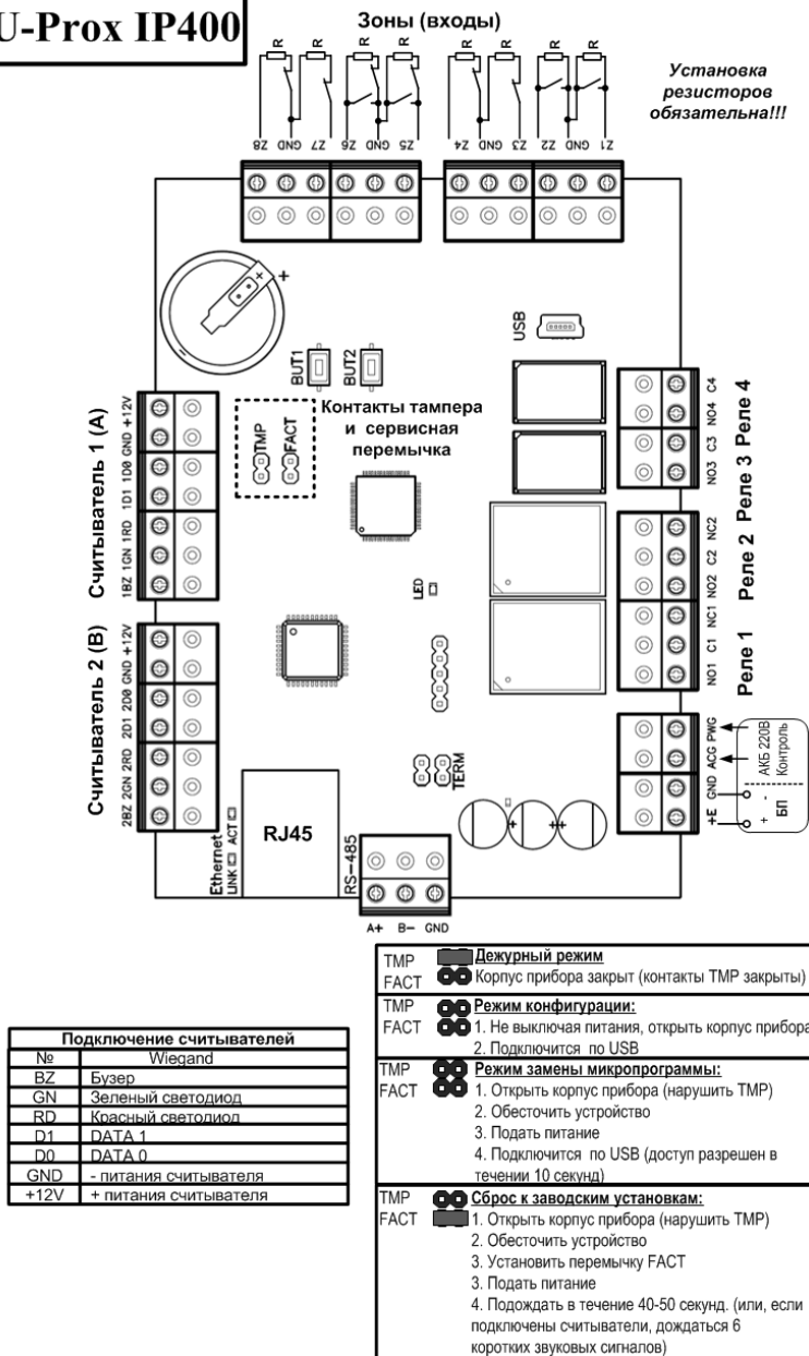
Рис. 2. Внешний вид платы контроллера
