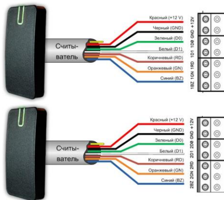
Рис.11. Подключение считывателей
