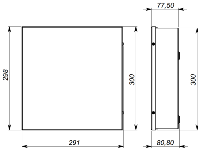
Рис 9. Габаритные размеры
